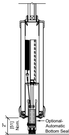
Optional Automatic Bottom Seal
